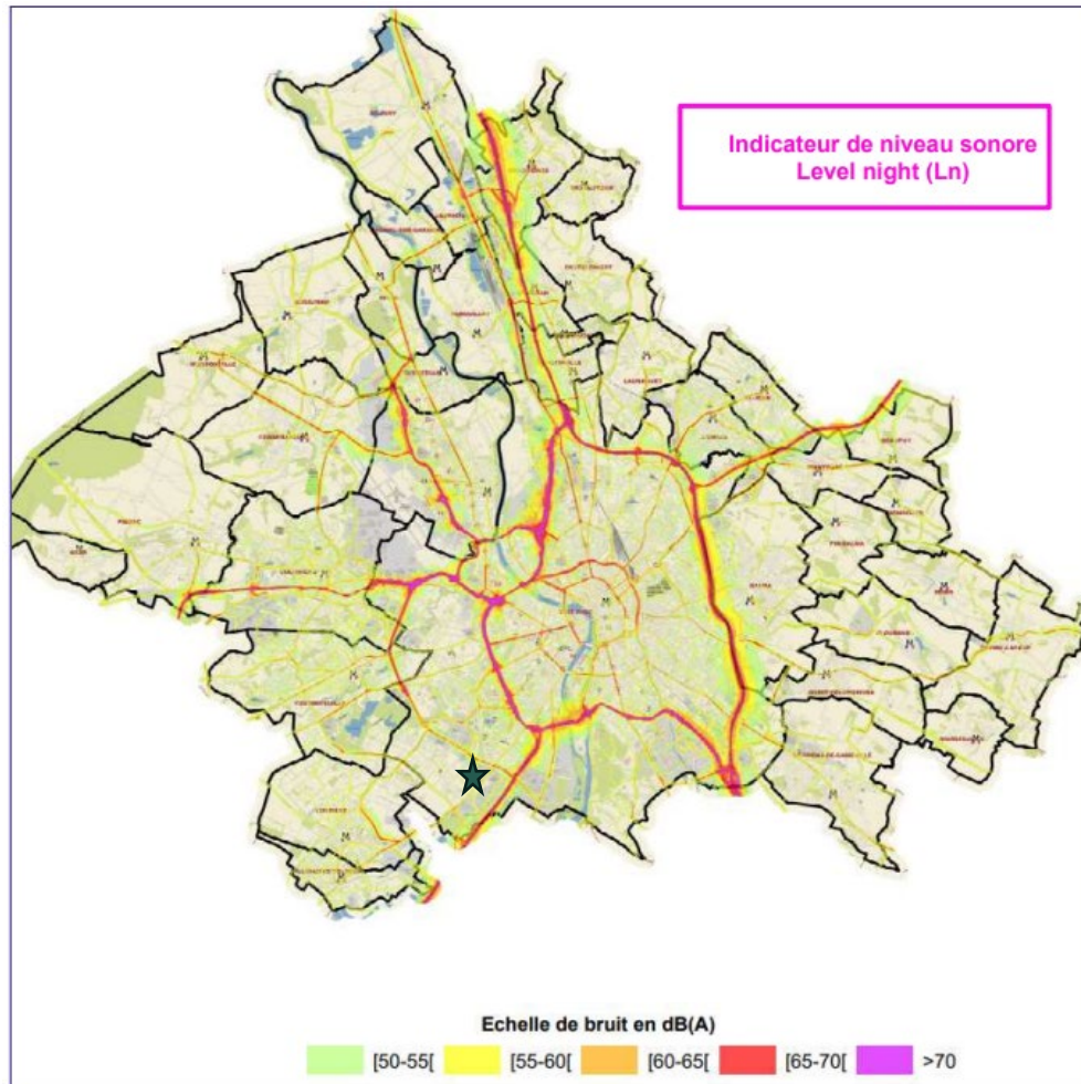
Bruit routier niveau nuit (source: projet de plan de prévention du bruit)
