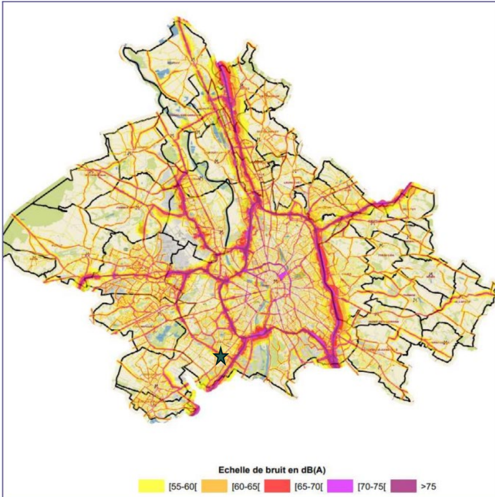
Bruit routier niveau moyen (source: projet de plan de prévention du bruit)
